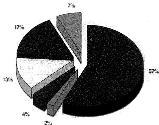
COMPOSIZIONE IMPIEGHI (QUOTE PERCENTUALI AL 31/12/99)
